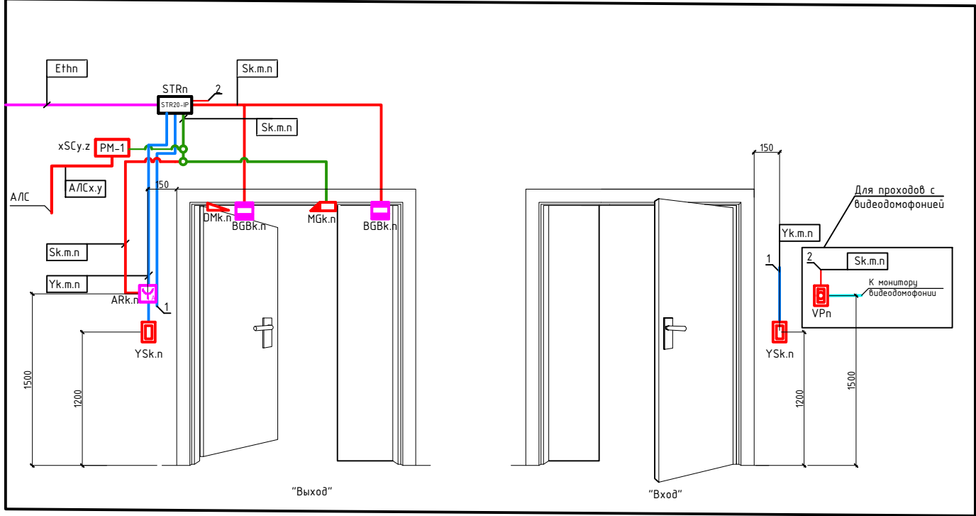
ТД Типовая точка доступа "Считыватель + Считыватель" для полуторных дверей
