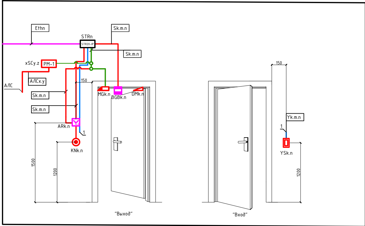
ТД Типовое решение по организации зоны доступа "Считыватель + Кнопка"
